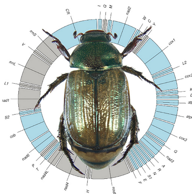
Esemplare di Mimela junii , con il suo genoma mitocondriale.
